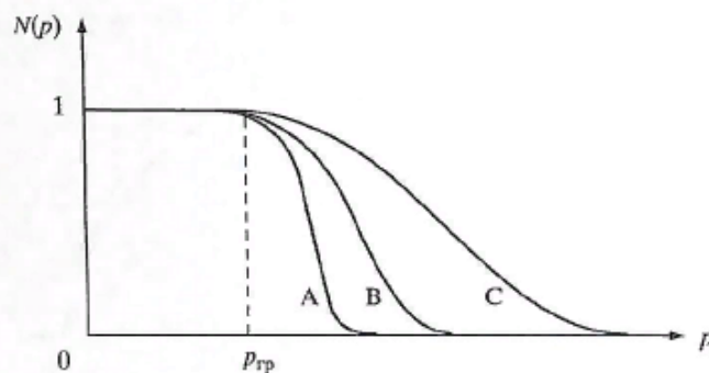
Рис. 3. Различные виды зависимости населенности от цены, даваемые формулой (4). Отношение предельной цены к граничной для кривых A, B и C равно соответственно 1,5; 2 и 3
