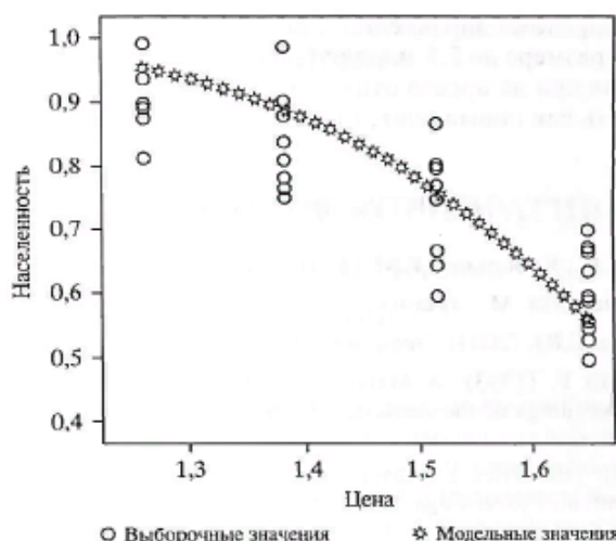
Рис. 4. Пример соответствия между выборочными значениями населенности и видом модельной зависимости, описываемой формулой (4)
